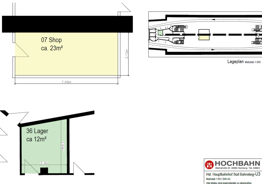
Abbildung 7: Grundriss und Lageplan der Ladenfläche
