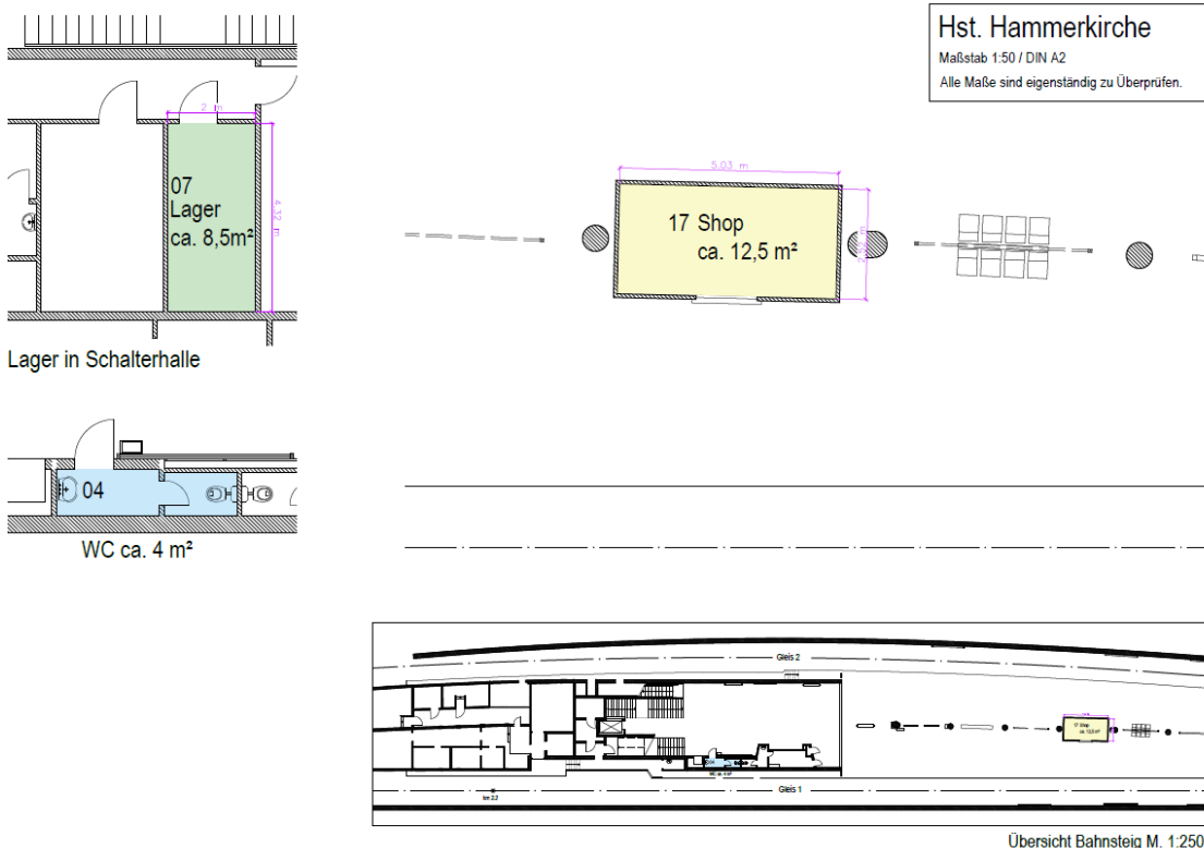
Abbildung 5: Grundriss Ladenfläche inkl. Lager
